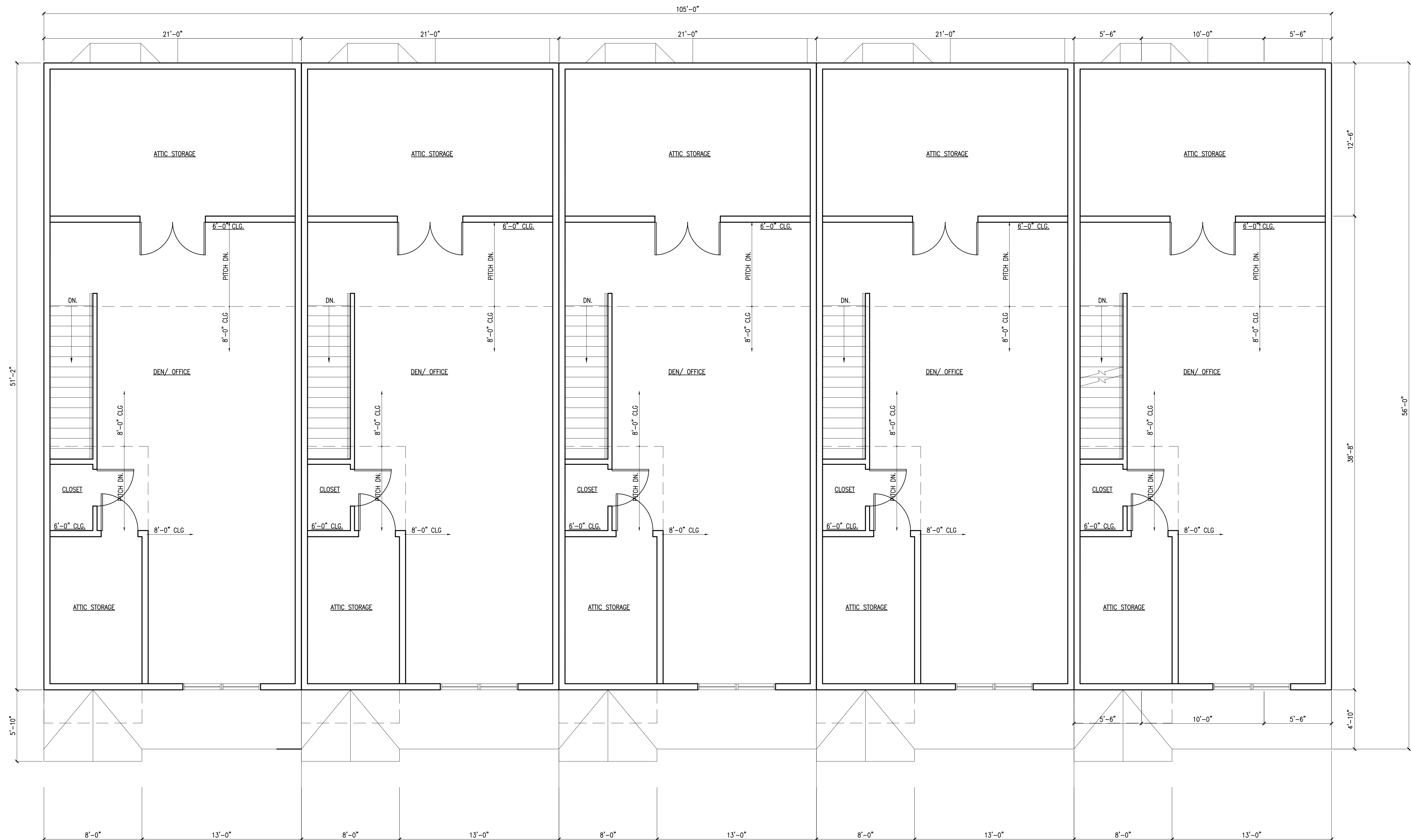
ATTIC SCALE: 1/4"=1'-0"
